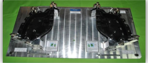
CF Rahmen Griffmulde hinten links/rechts G12
