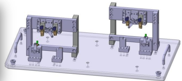
CF Schalterblende SPA BFS & FS vorne LL/RL
